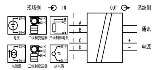
UW5261 通用模拟量输入模块隔离电气原理图
