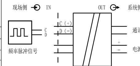
UW5264 脉冲量输入模块隔离电气原理图
