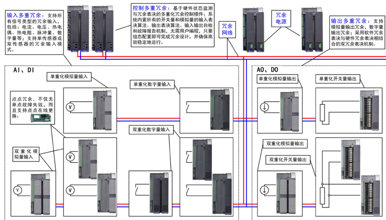
UW500a集散控制系统冗余结构图
