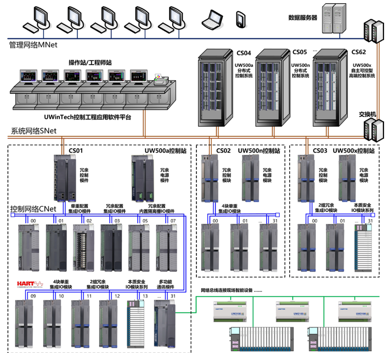
UW500集散控制系统系统结构图
