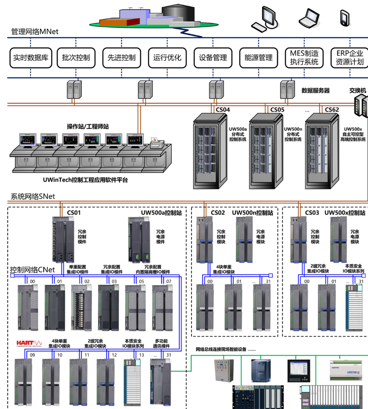
UW500集散控制系统网络结构图
