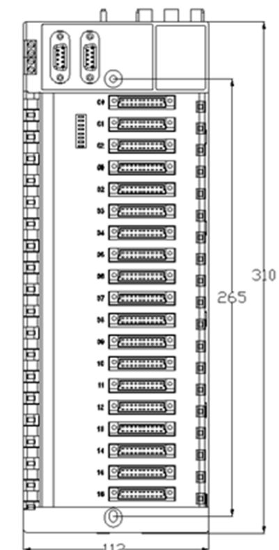
UW5850 底座安装尺寸图
