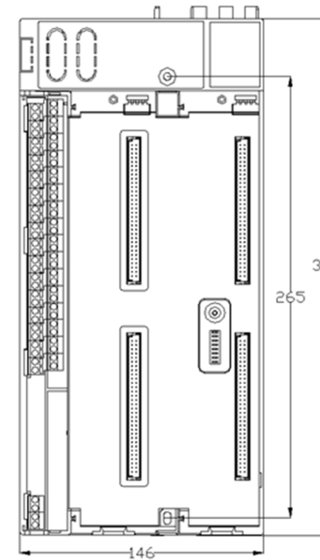
UW500a 底座安装尺寸图
