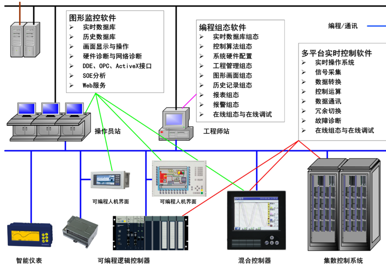
UWinTech 系统软件构成图
