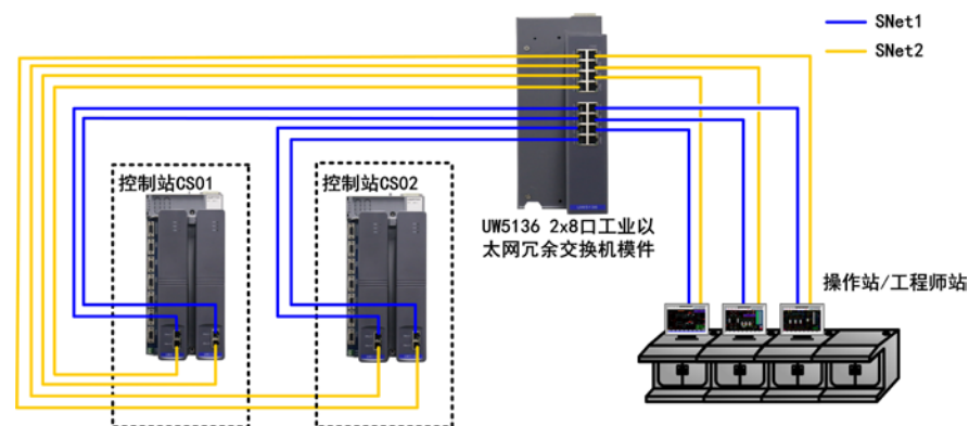
系统网络连接示例图(控制站 *2、操作站 *3)
