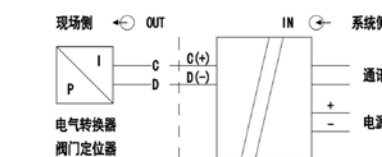
UW5266 模拟量输出模块隔离电气原理图
